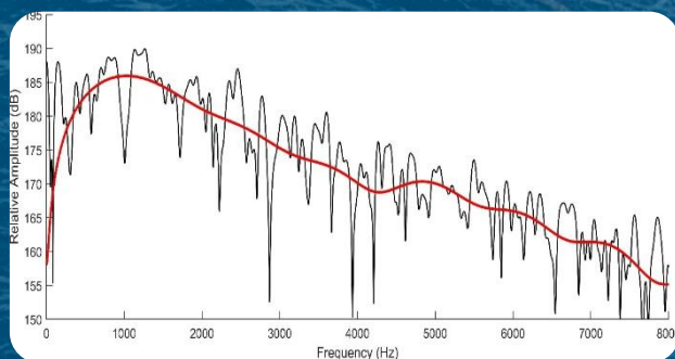
波形测试e-Boomer 300S @1000J
